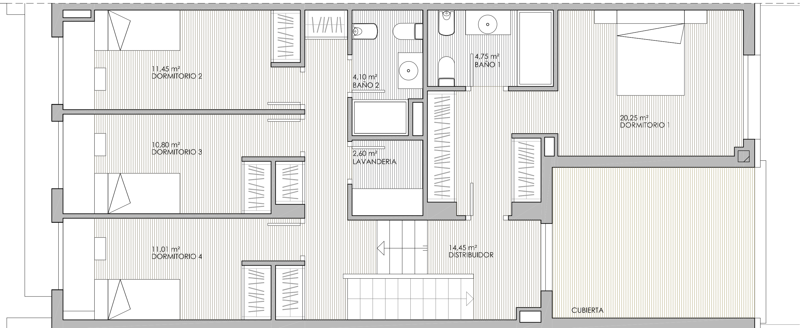
PLANTA PRIMERA
