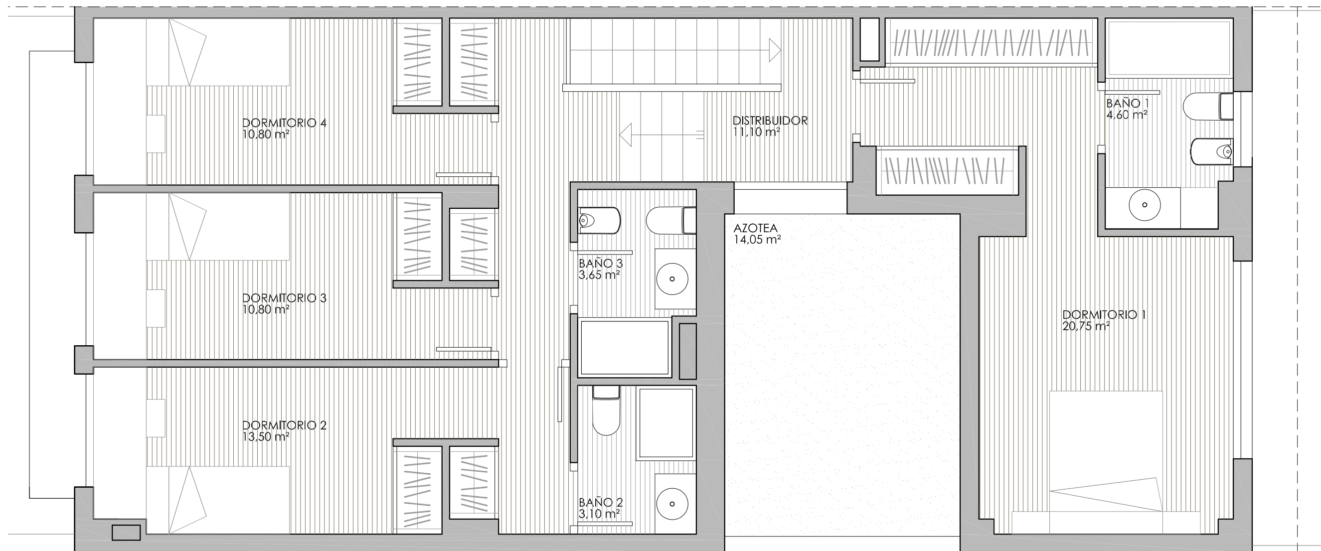
PLANTA PRIMERA
