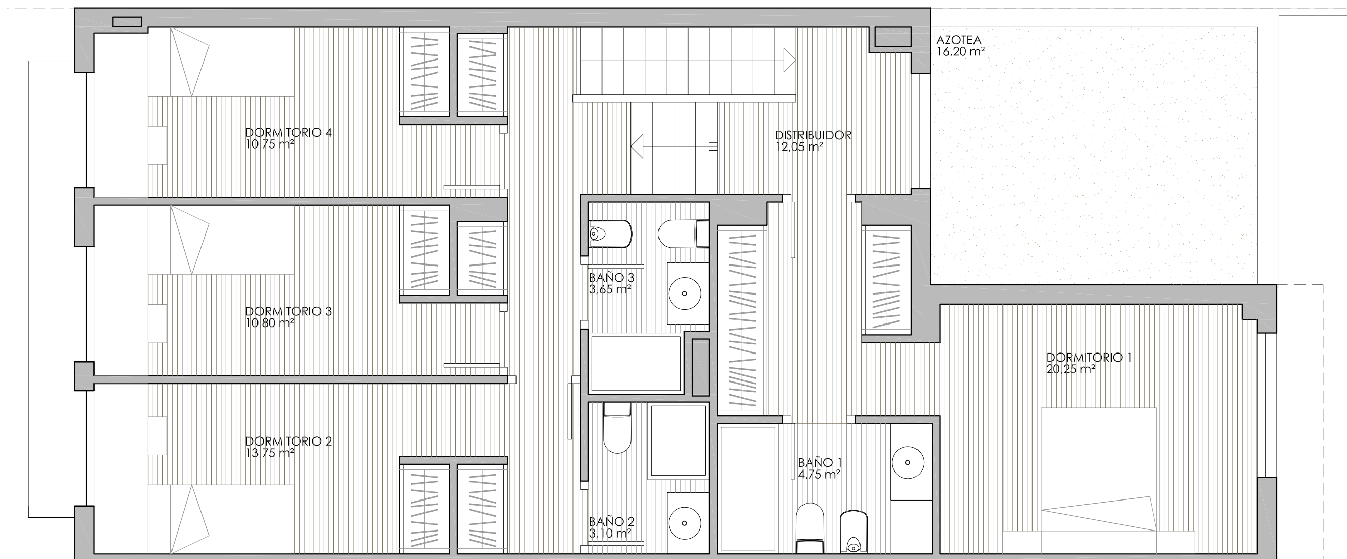
PLANTA PRIMERA
