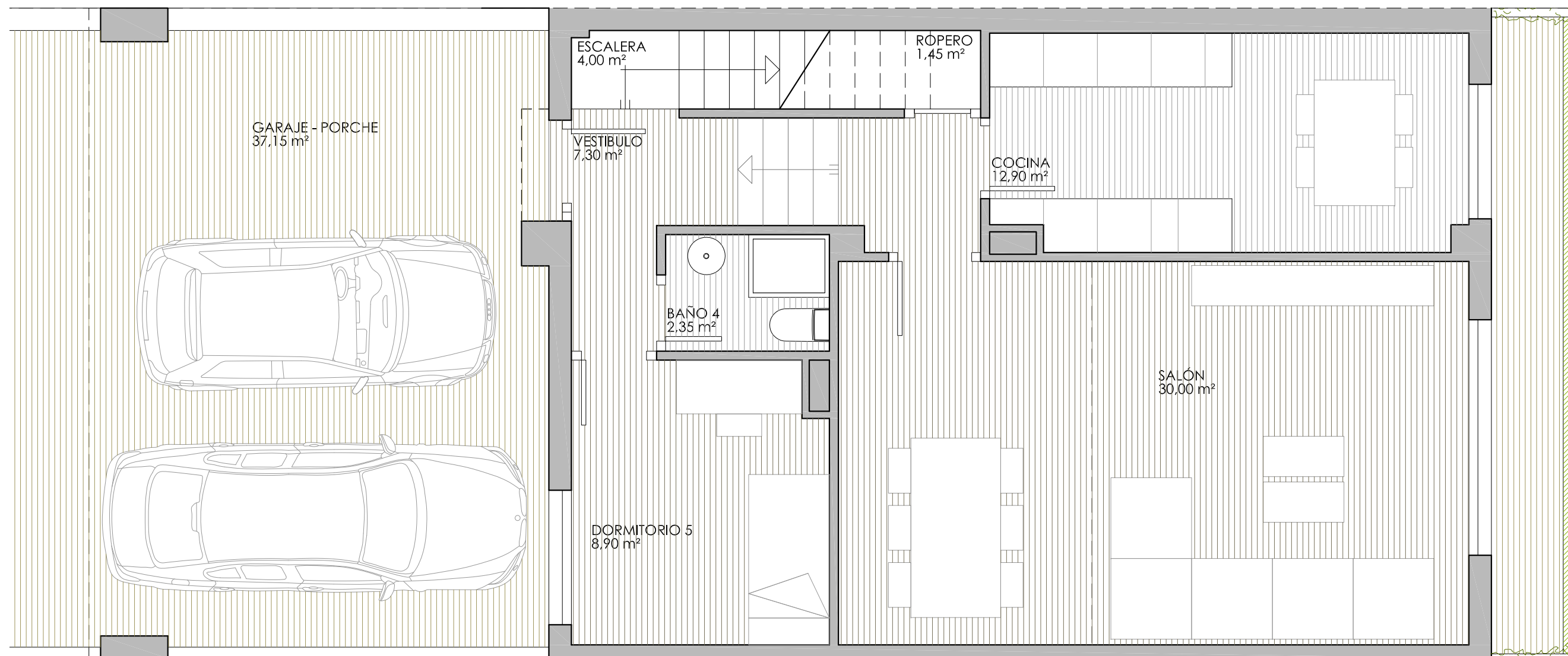
PLANTA BAJA
