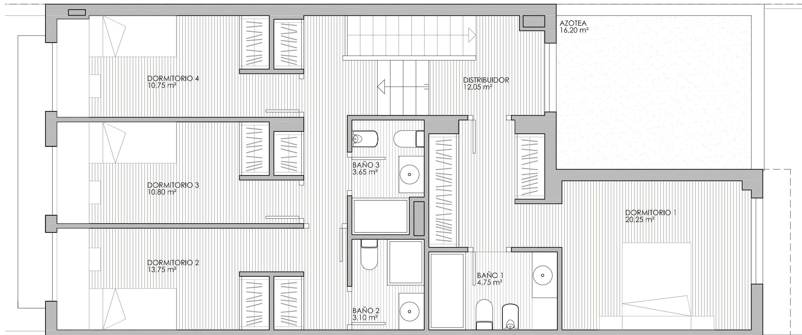
PLANTA PRIMERA
